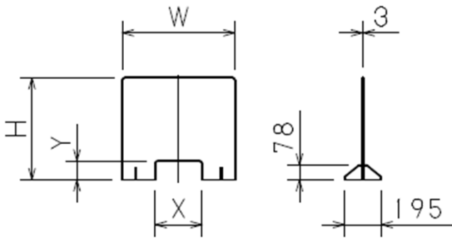
製品寸法
